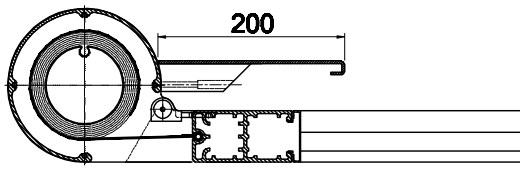
TETTUCCIO - COVERING - TOITURE
