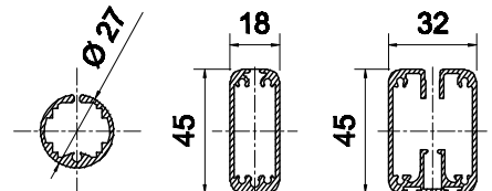
TERMINALE HEM BAR - BARRE FINALE
