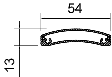
TERMINALE HEM BAR BARRE FINALE
