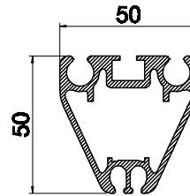
Profilo porta telo A
