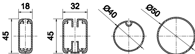
TERMINALE - HEM BAR - BARRE FINALE
