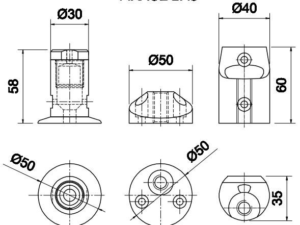
TENDIFUNE INFERIORE LOWER BRACKET FIXAGE BAS
