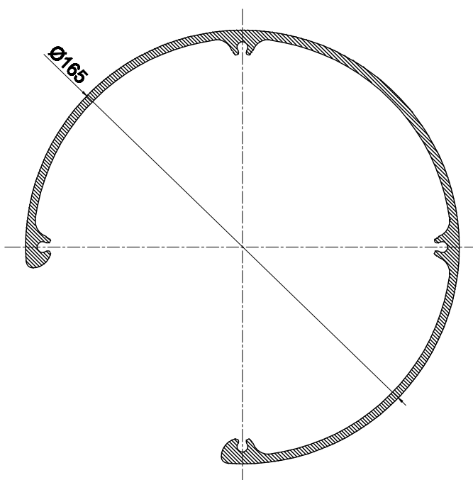
CASSONETTO - HEAD BOX - CAISSON
